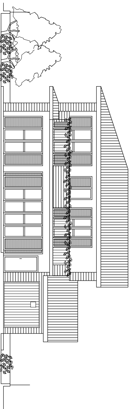
Prospetto sud
